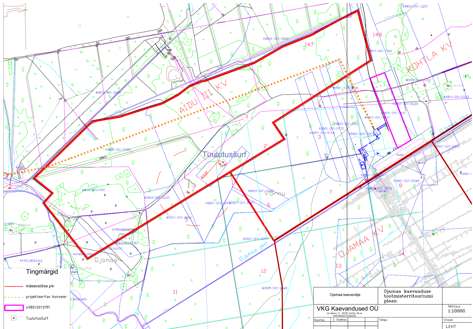
Skeem 4. VKG Kaevandused OÜ planeeritava lintkonveieri asukoha trass (Uus-Kiviõli konveier).
