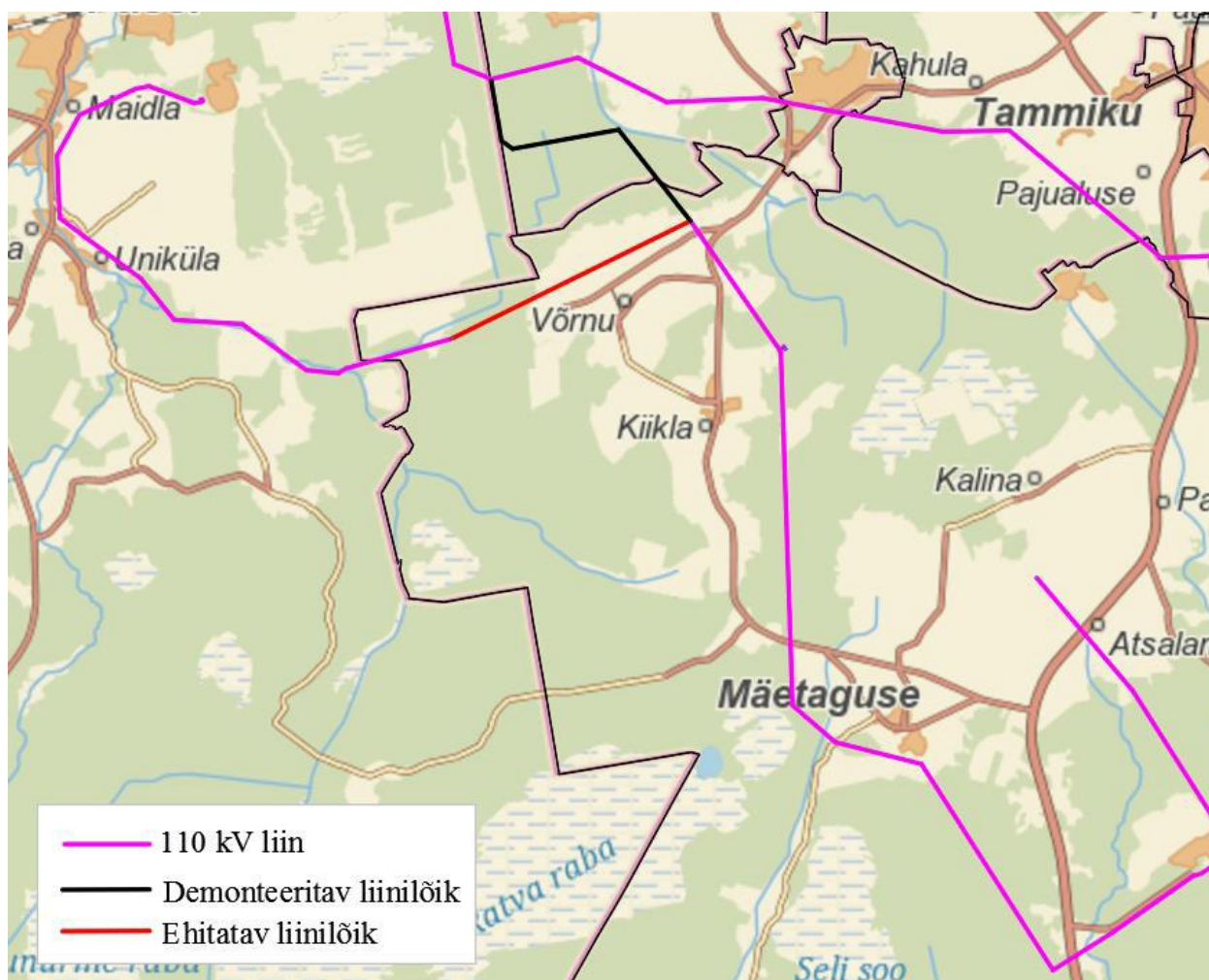
Skeem 5. Liini L138A ümberehitus.
